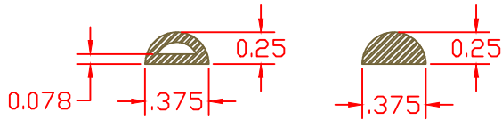
GASKET MS27684-27
